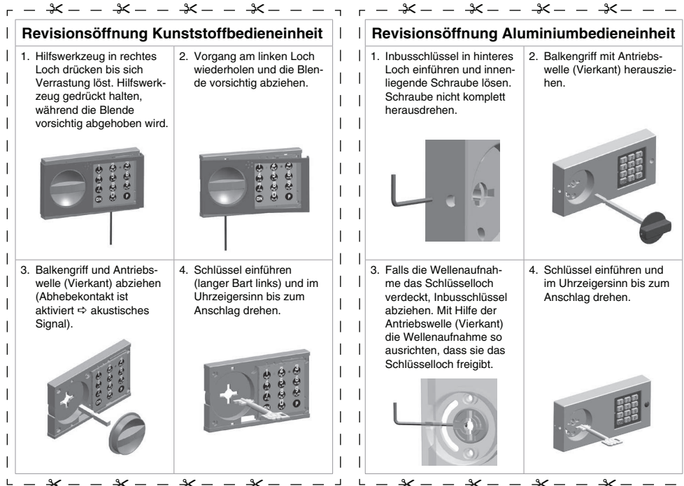
Abb. 6: Kunststoffbedieneinheit
